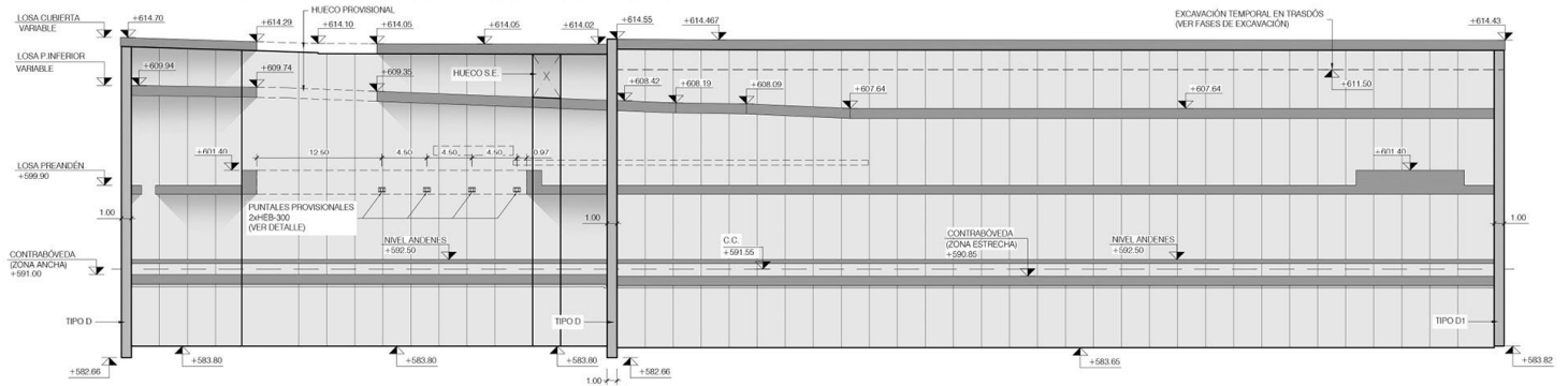
Recálculo y análisis de deformaciones en la Estación Conde de Casal y recálculo de pantallas y losas en la Estación Comillas
