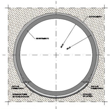
FASE 6: SECCIÓN FINAL Escala: 1:50 NOTA: TODAS LAS COTAS ESTÁN EN METROS
