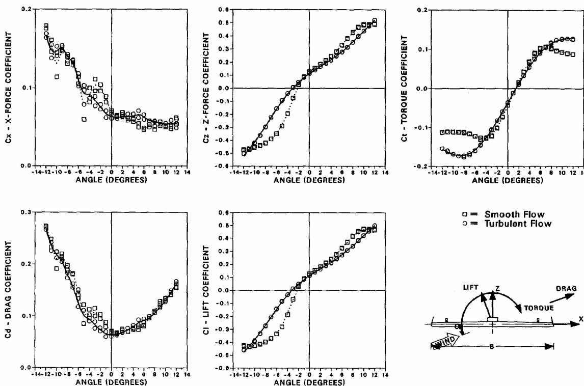
Figura 9. Coeficientes de empuje estático.
