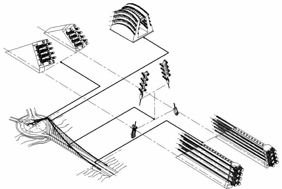
Figura 4. Sistema de suspensión.
