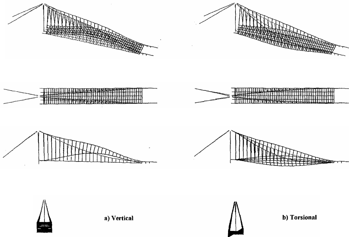
Figura 8. Modos de vibración.
