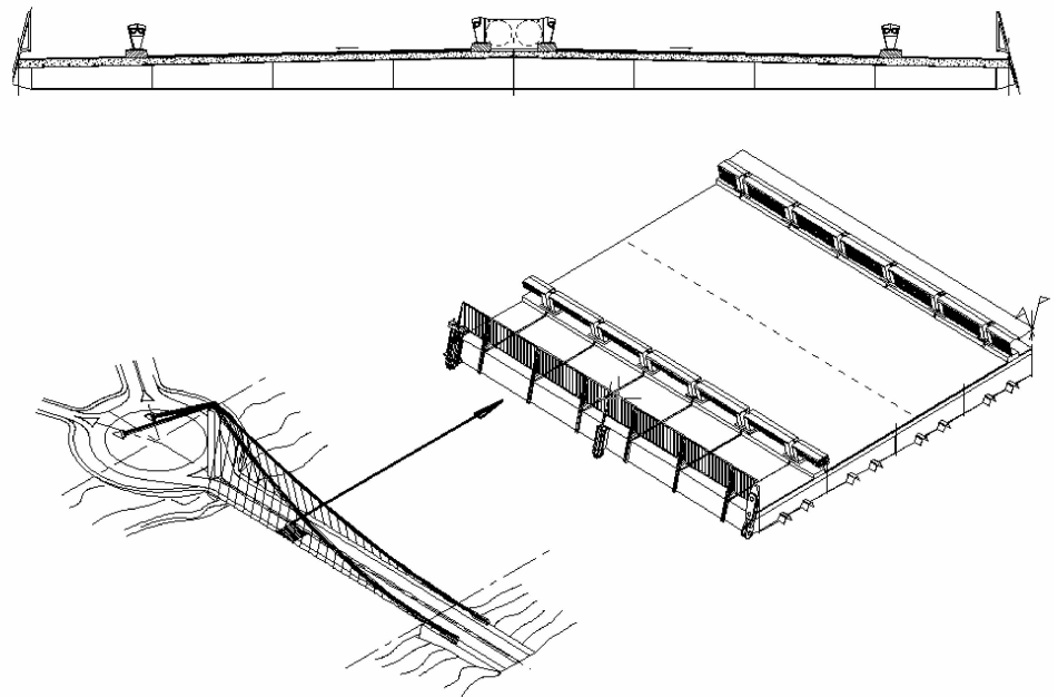
Figura 5. Sección transversal.
