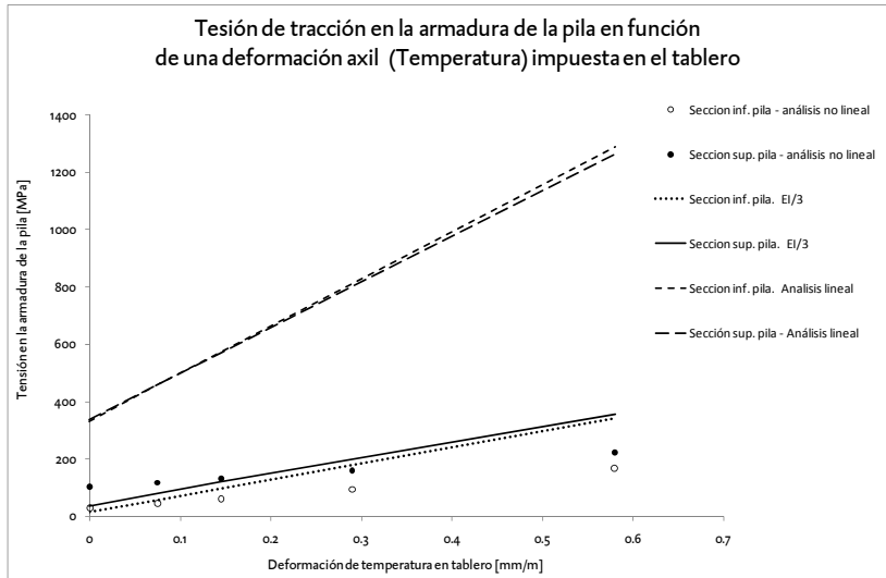
Fig 6. Tensión de tracción en la armadura de las pilas en función de la deformación impuesta en el tablero (cálculo lineal, cálculo con rigidez a flexión reducida y análisis no lineal)
