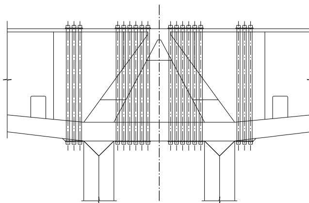
Fig. 13. Pretensado vertical en la sección de apoyos para compensar la pérdida de armadura en las células triangulares por la ejecución de taladros necesarios para anclar el pretensado exterior.
