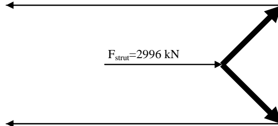
Fig. 9. Modelo de bielas y tirantes que muestra cómo la componente horizontal de los jalcónes puede ser resistida por la armadura de la estructura existente mediante su difusión en un ancho importante. Para equilibrar los nudos exteriores del modelo, es necesario contar con una armadura longitudinal (paralela al eje de la estructura).
