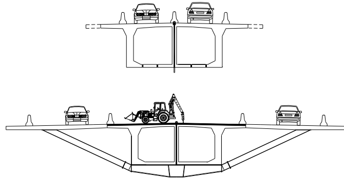
Fig. 8 – Dos fases del proceso constructivo que permite la ejecución de la ampliación de la losa y la conexión de esta ampliación al tablero existente. El tráfico se mantiene durante todo el proceso.
