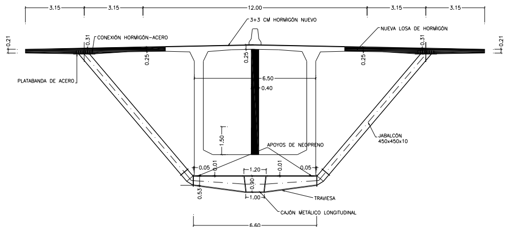
Figura 2 – Concepción estructural de los elementos de refuerzo del tablero (sección transversal)
